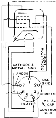
TRIODE-HEXODES
