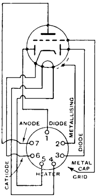
DOUBLE DIODE TRIODES MHD4 DH3 DH30
